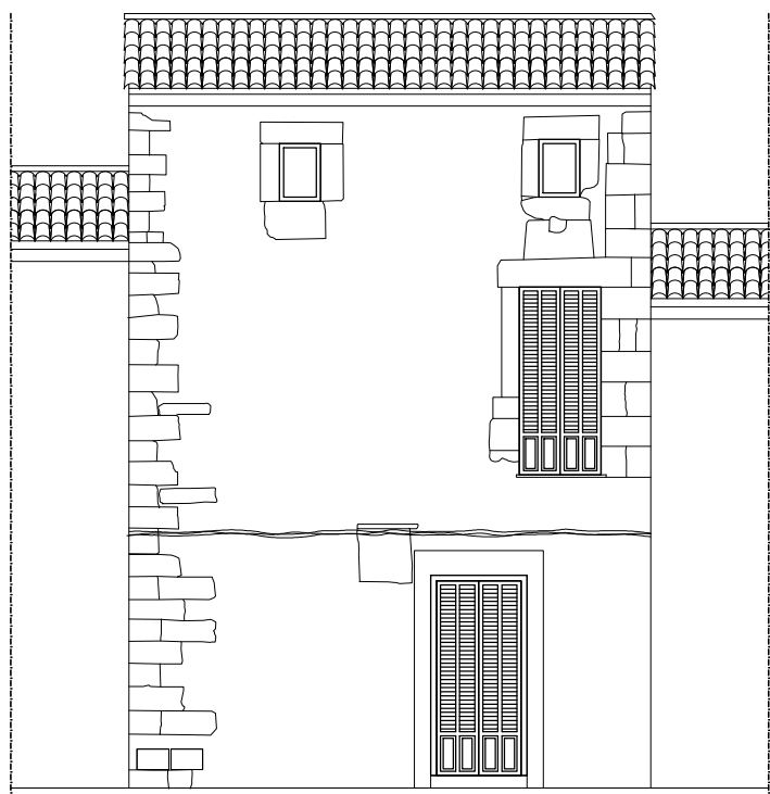
ALZADO PRINCIPAL E 1:100
